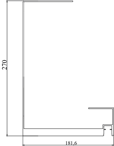
TRAVE MOTORE
