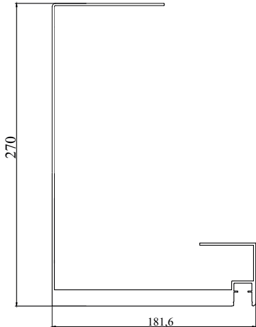
GRONDA
