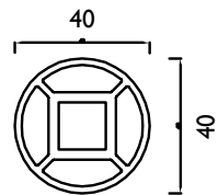
PROFILO TRASMISSIONE
