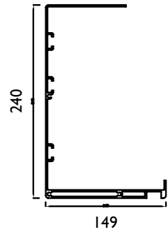
PROFILO TRASMISSIONE
