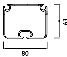
PROFILO TELO
